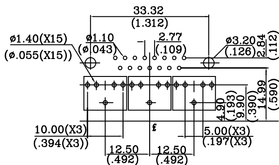
P.C.B LAYOUT
