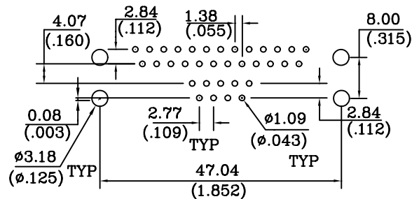
P.C.B LAYOUT
