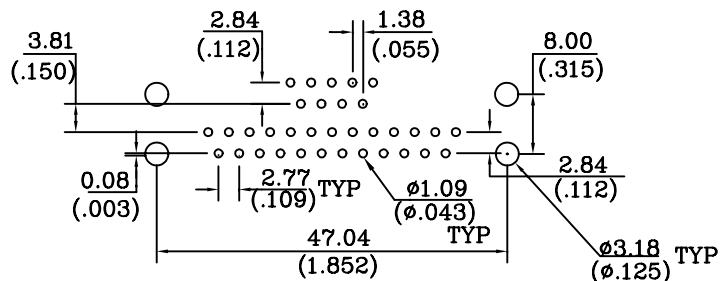
P.C.B LAYOUT
